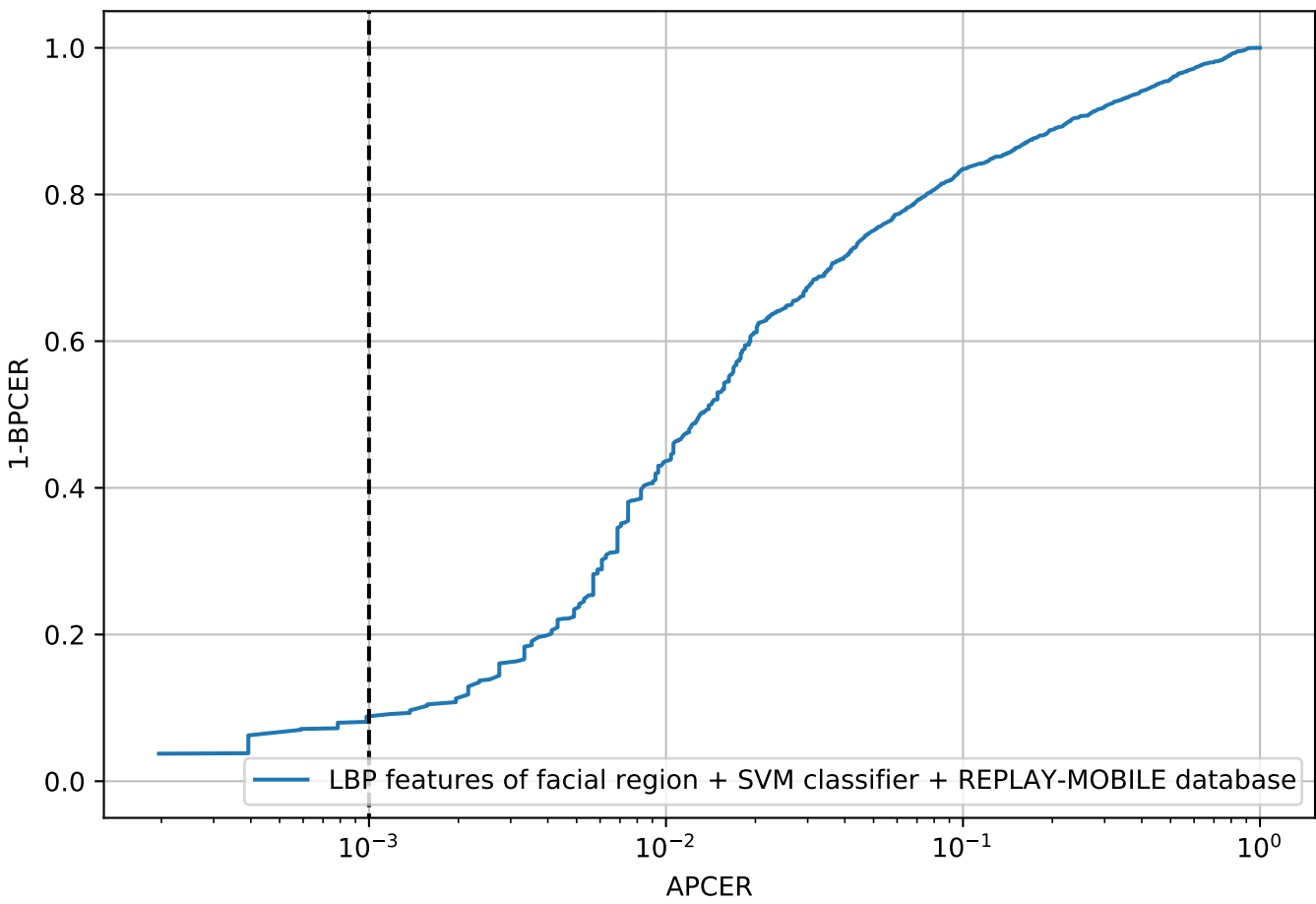
ROC dev.
