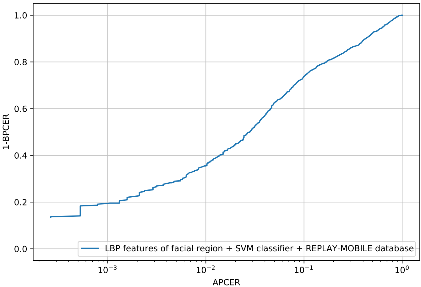
ROC eval.
