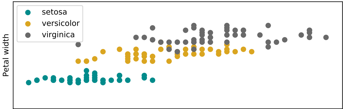
Raw fetures
