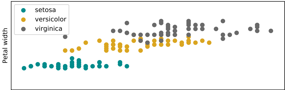
Raw fetures
