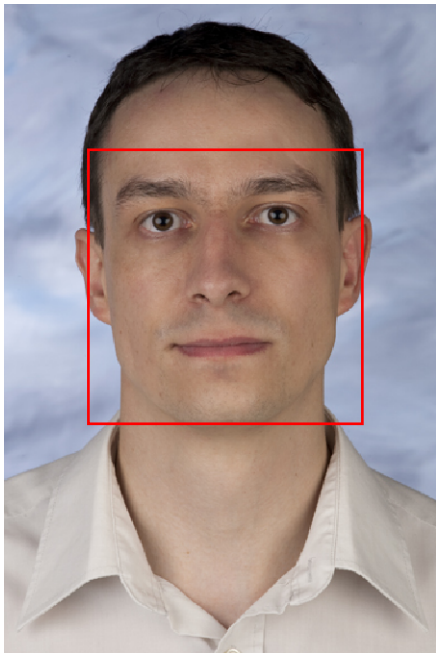
bob.ip.dlib
