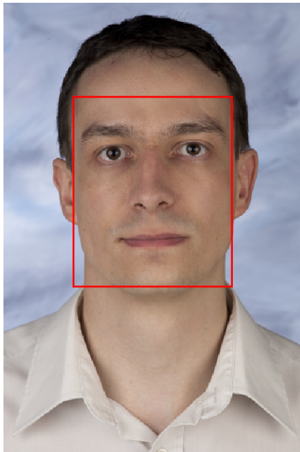
bob.ip.facedetect
