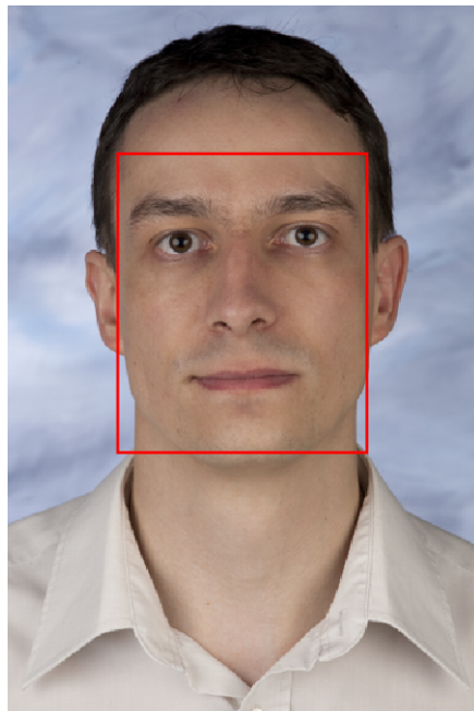
bob.ip.facedetect
